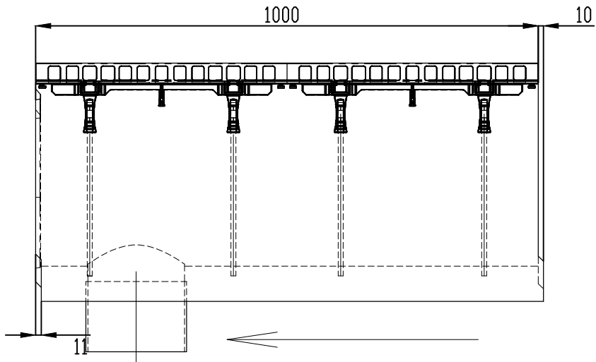
Арт. 40730171 BGM Массивный лоток DN 300, № 5-0, с вертикальным водосливом без уклона, кл. А В С D E F.
